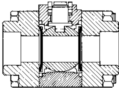
Kulový uzávěr
