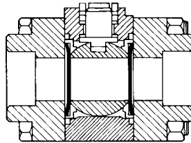
Kulový uzávěr
