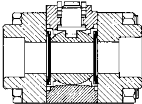
Kogelventiel
