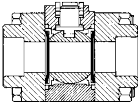
Zawór kulowy
