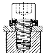
Przed zaciśnięciem
