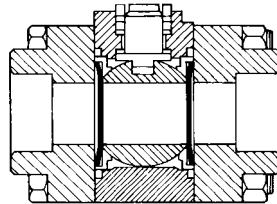
Zawór kulowy
