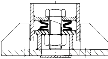
Amortyzacja wstrząsów
