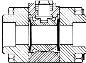
Válvula de bola
