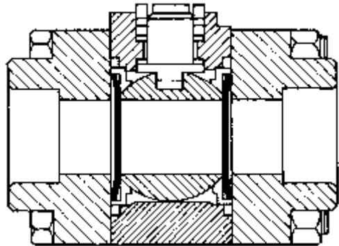
Valvă sferică
