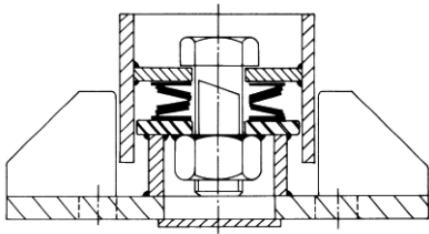
Preluare șocuri
