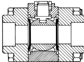
Valvă sferică
